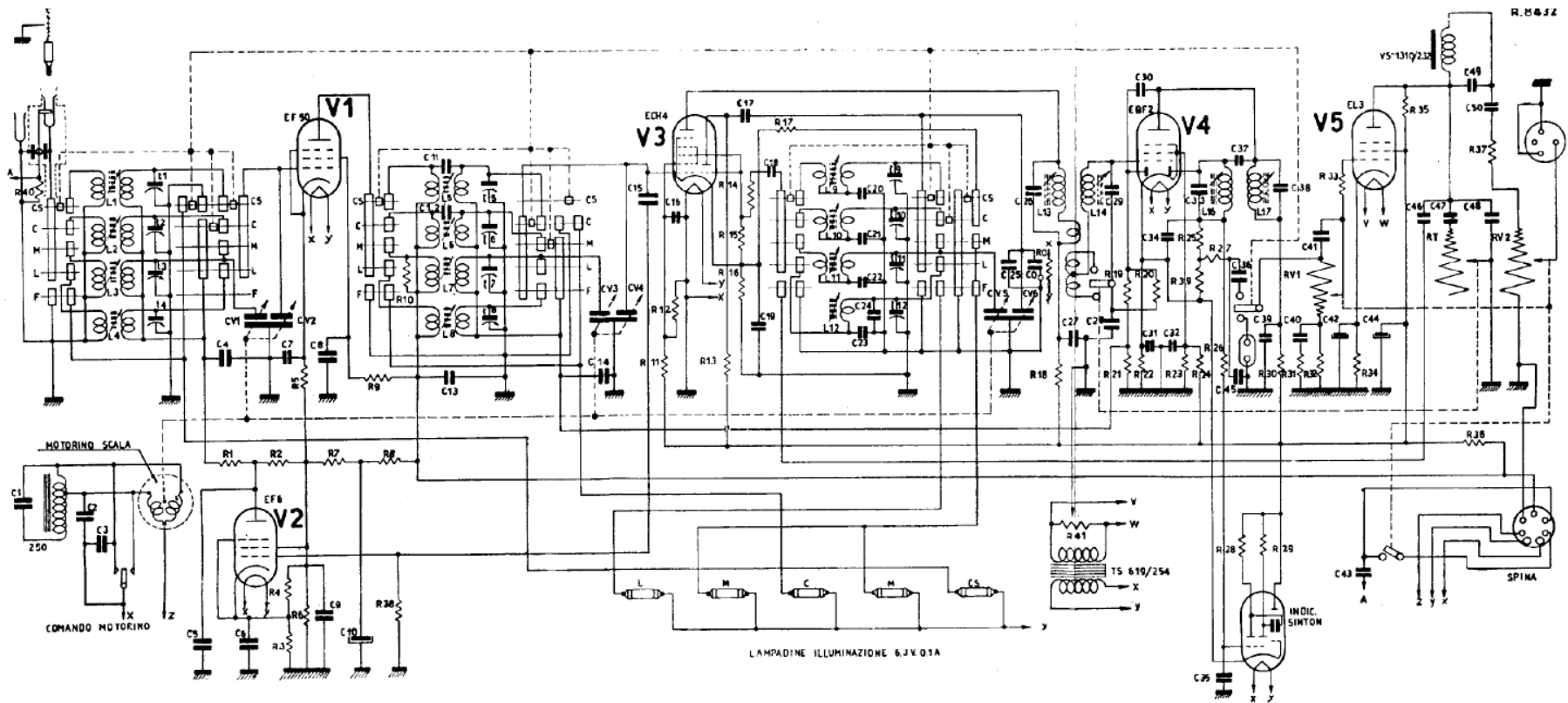
PHONOLA RADIO. — Mod. 814. — Valvole, condensatori e resistenze v. Tabelle. — MF. 470 kHz. — Produzione 1943.
